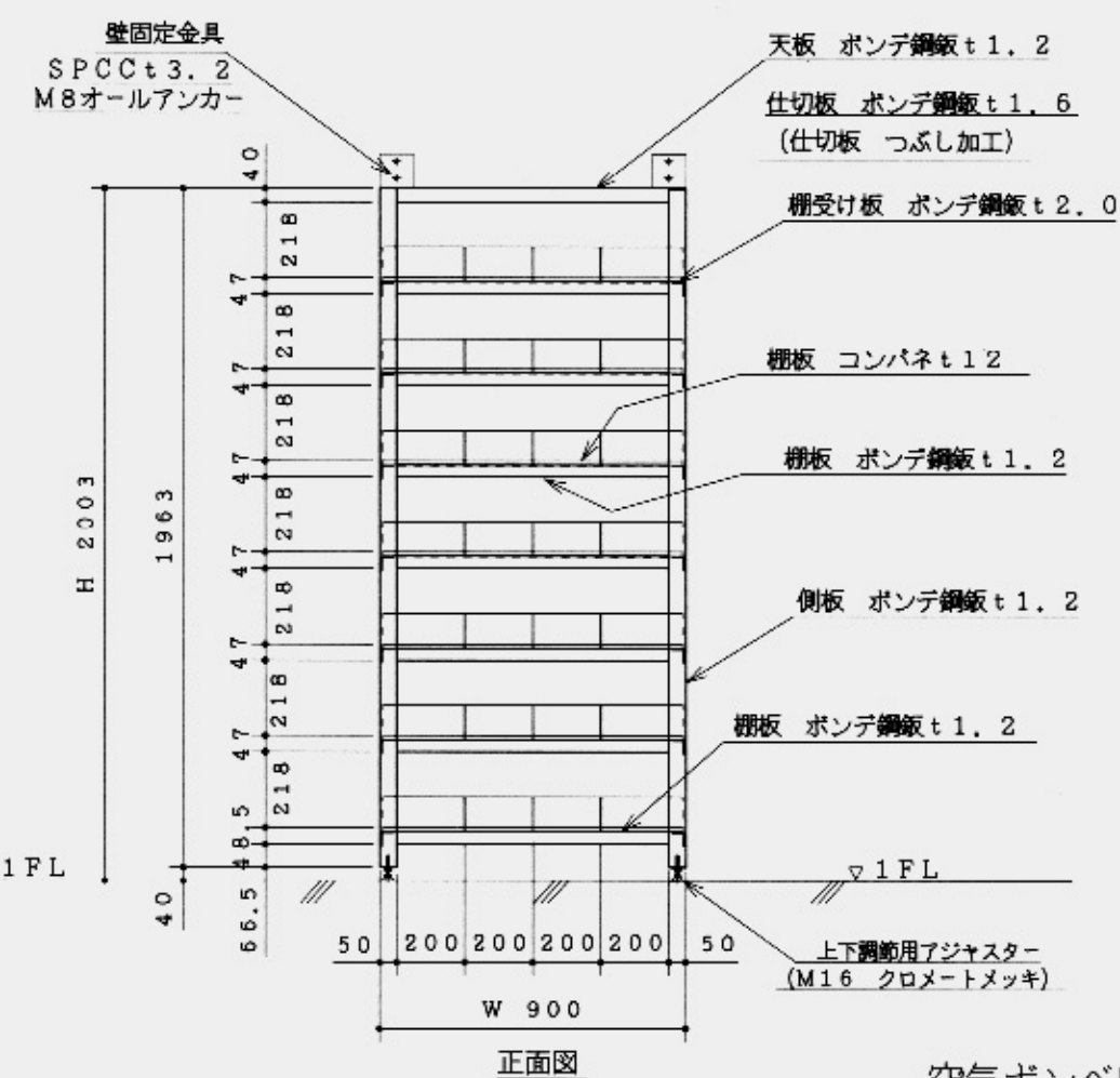
空気ポンベ収納棚 詳細図
