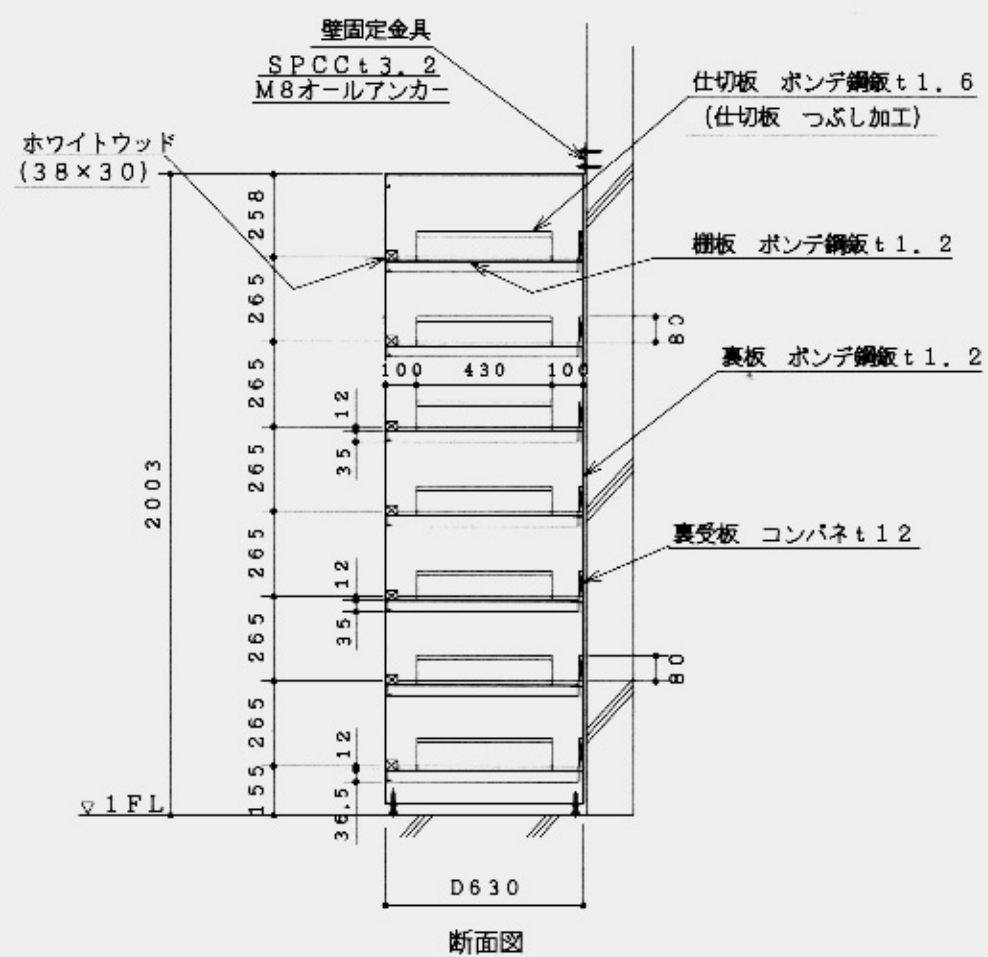
空気ポンベ収納棚 詳細図
