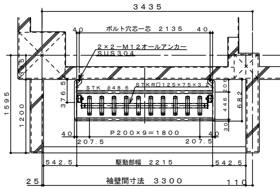
ハンガー及びレールブラケット平面
