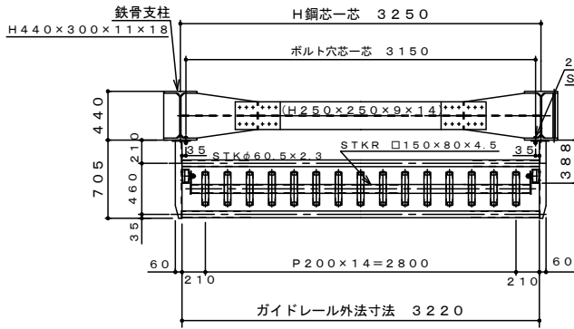
ハンガー及びレールブラケット平面
